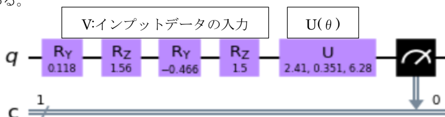
図 21 1量子ビット量子回路
