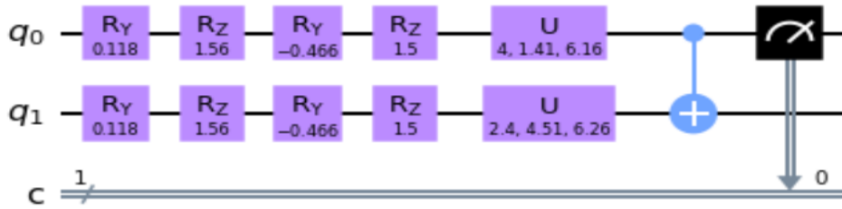
図22 2量子ビット量子回路
